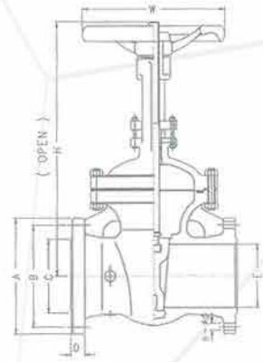
ANSI 300/JIS 20K
