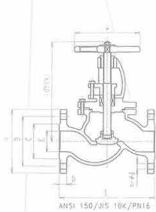
ANSI 150/JIS 10K/PN16
