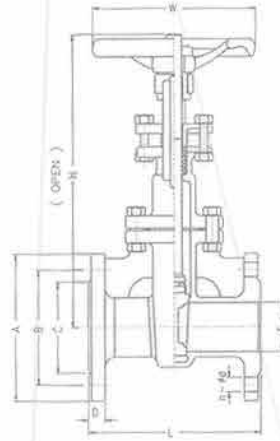
ANSI 150/JIS 10K/PN10
