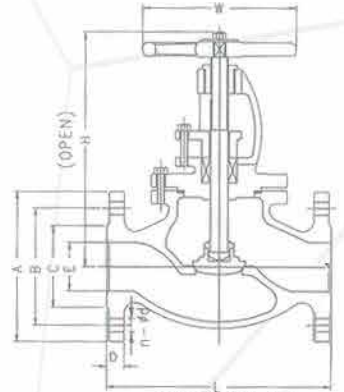
ANSI 300/JIS 20K
